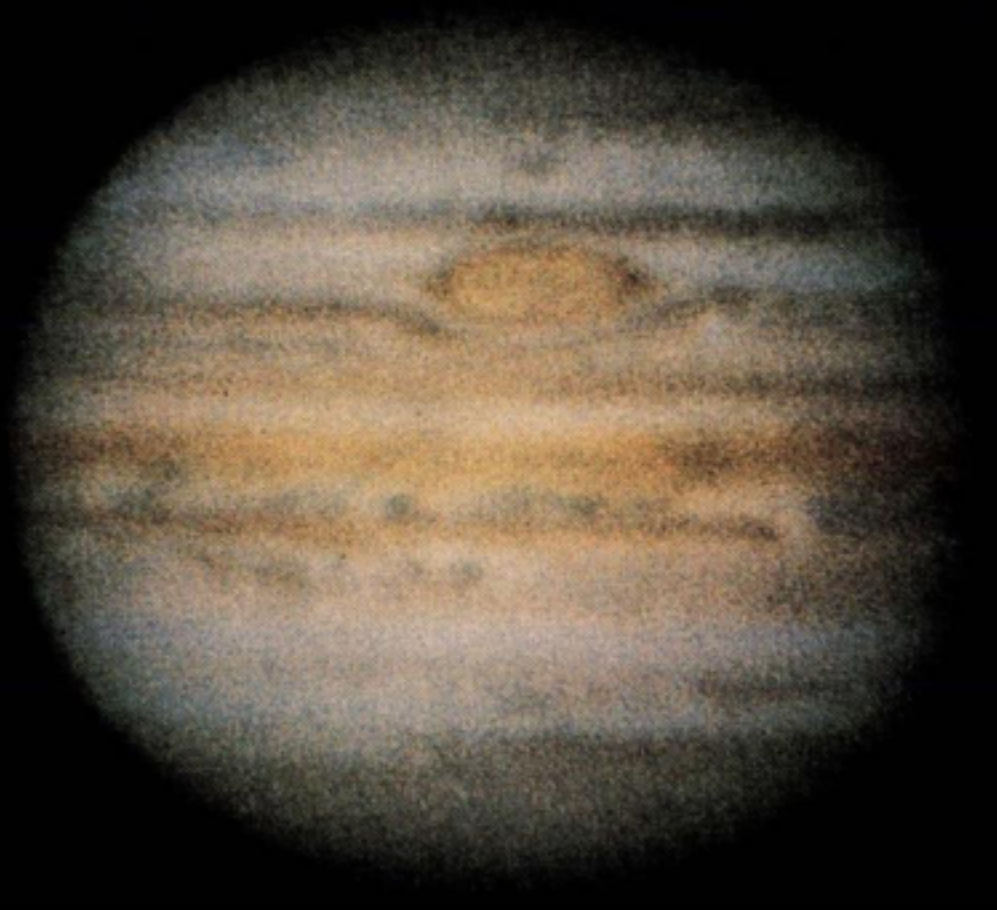
1968-05-18 LPL Univ.Arizona
