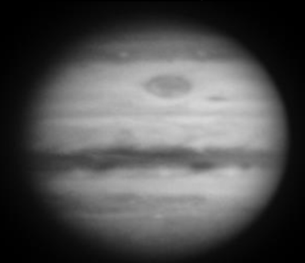
1989-09-28 I. Miyazaki
