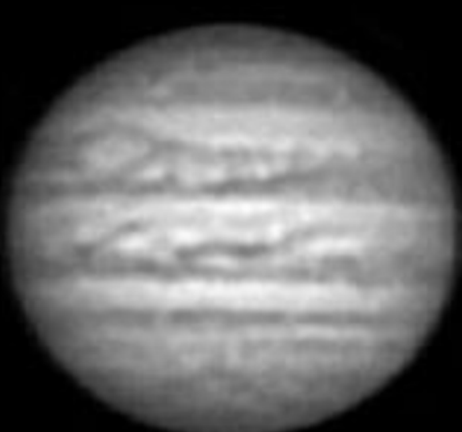
1998-08-27 D. Peach
