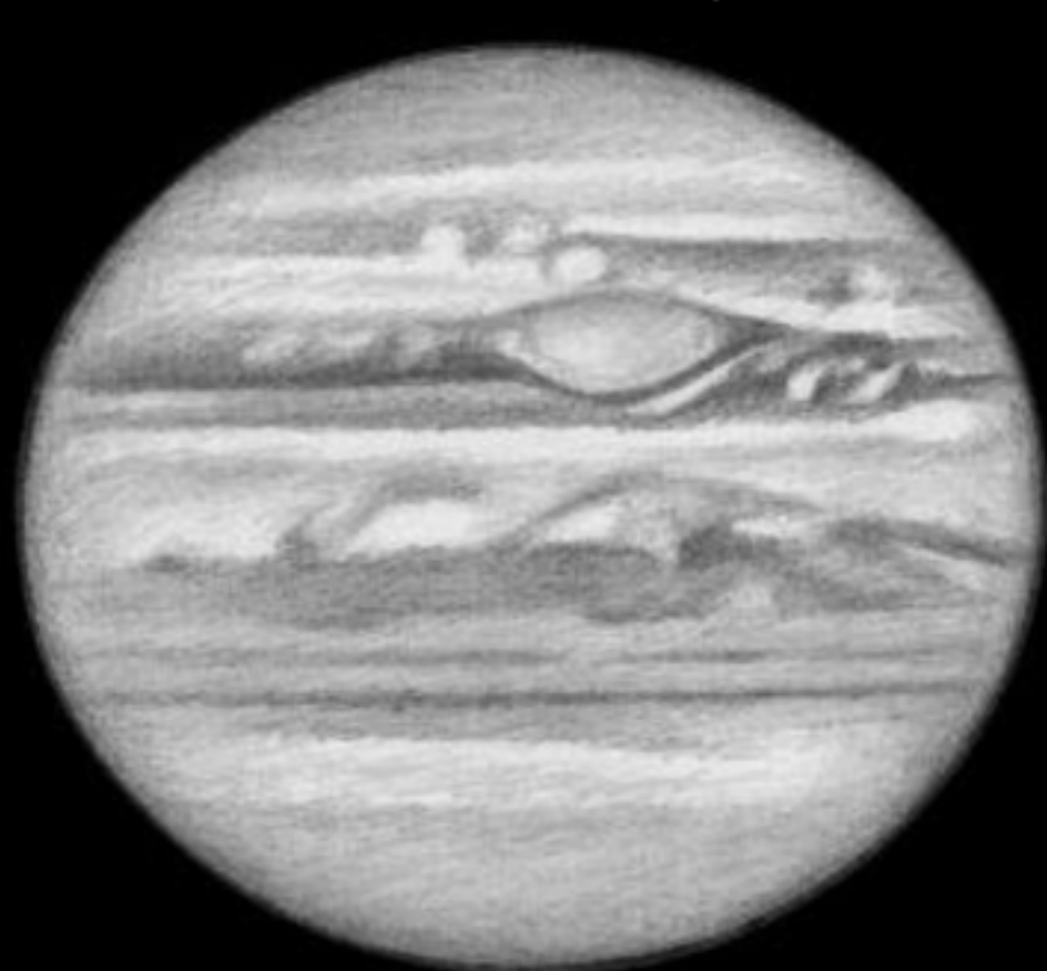
1985-05-25 I. Miyazaki
