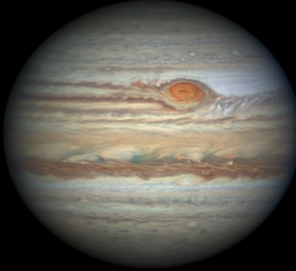
2019-05-26 C. Go
