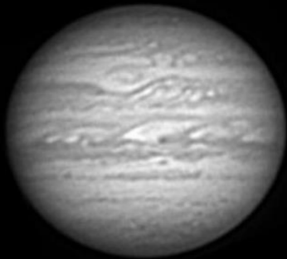
1999-10-06 D. Peach
