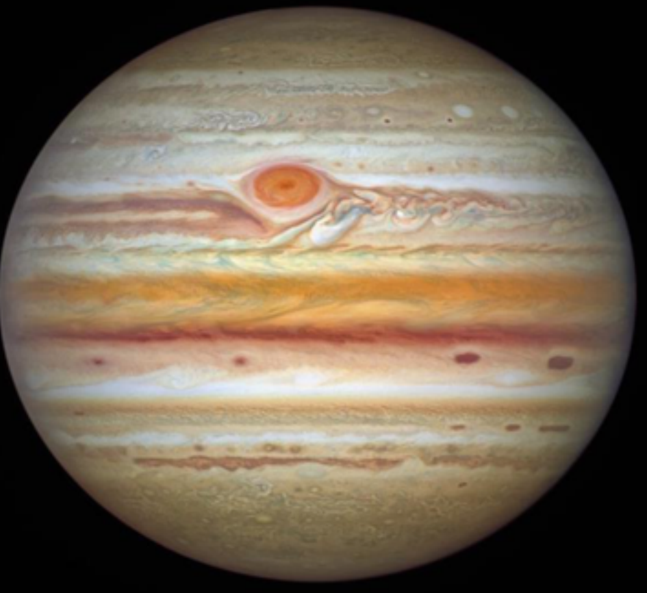
2021-09-04 HST
